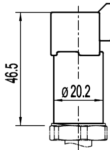
Deutsch connector
